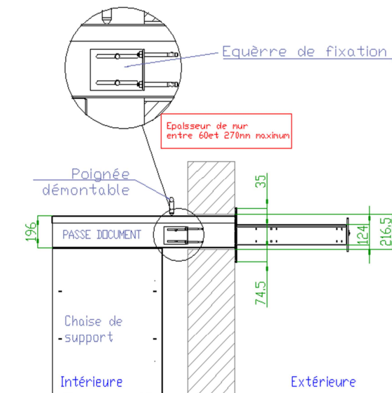
COUPE C-C
