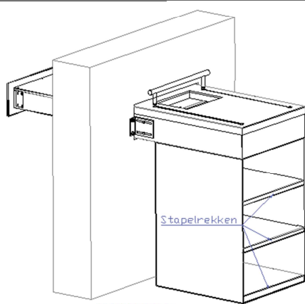
PERSPECTIEF
