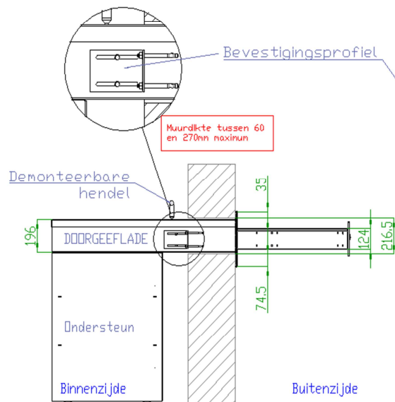
DOORSNEDE C-C
